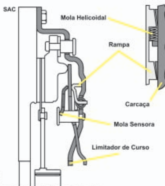
Disco desgastado
