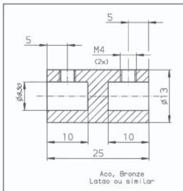
Detalle del prolongador
