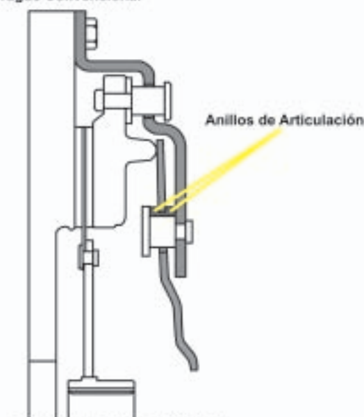
Embrague Convencional
