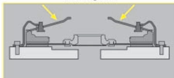
Diafragma con ángulo alterado
