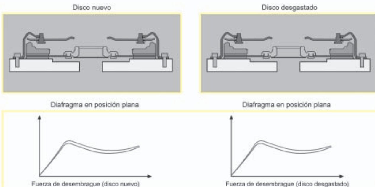
Fig. 4 - Embrague Auto-ajutable
