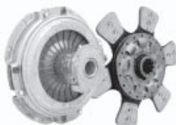
Membrana de 14" Ceramético
