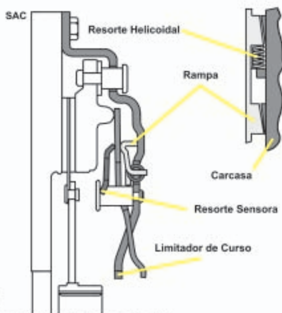
Fig. 3 Embrague Auto-ajutable
