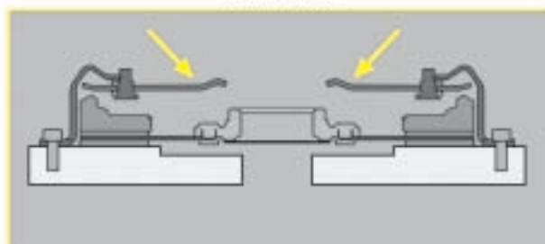
Diafragma en posición plana
