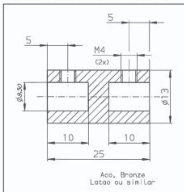
Detalhe do prolongador
