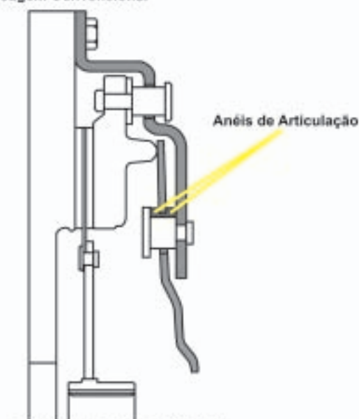
Embreagem Convencional
