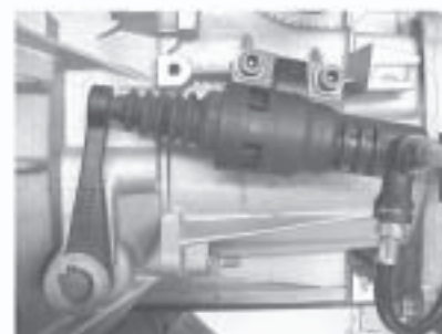
Fig. 08 Haste do Cilindro Escravo
