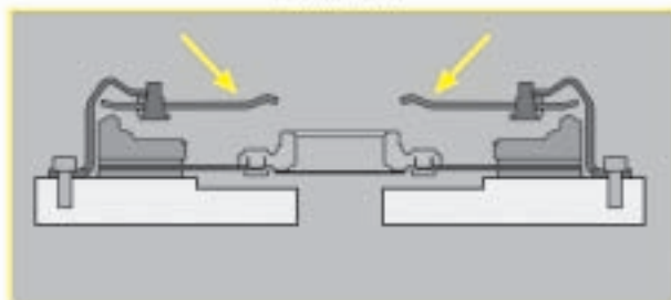
Diafragma na posição plana
